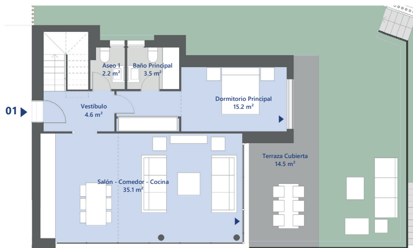
Planta baja
