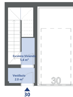
Planta sótano
