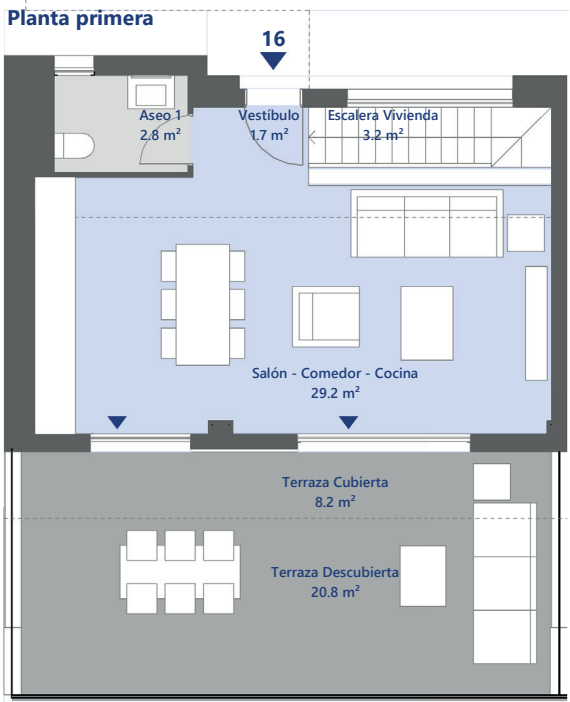
Planta primera
