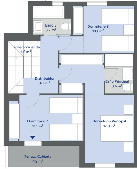
Planta primera
