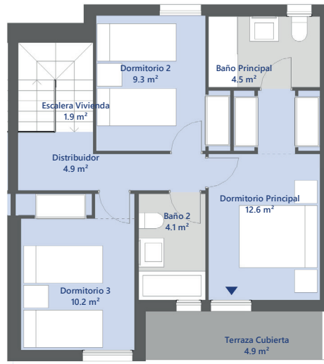
Planta primera
