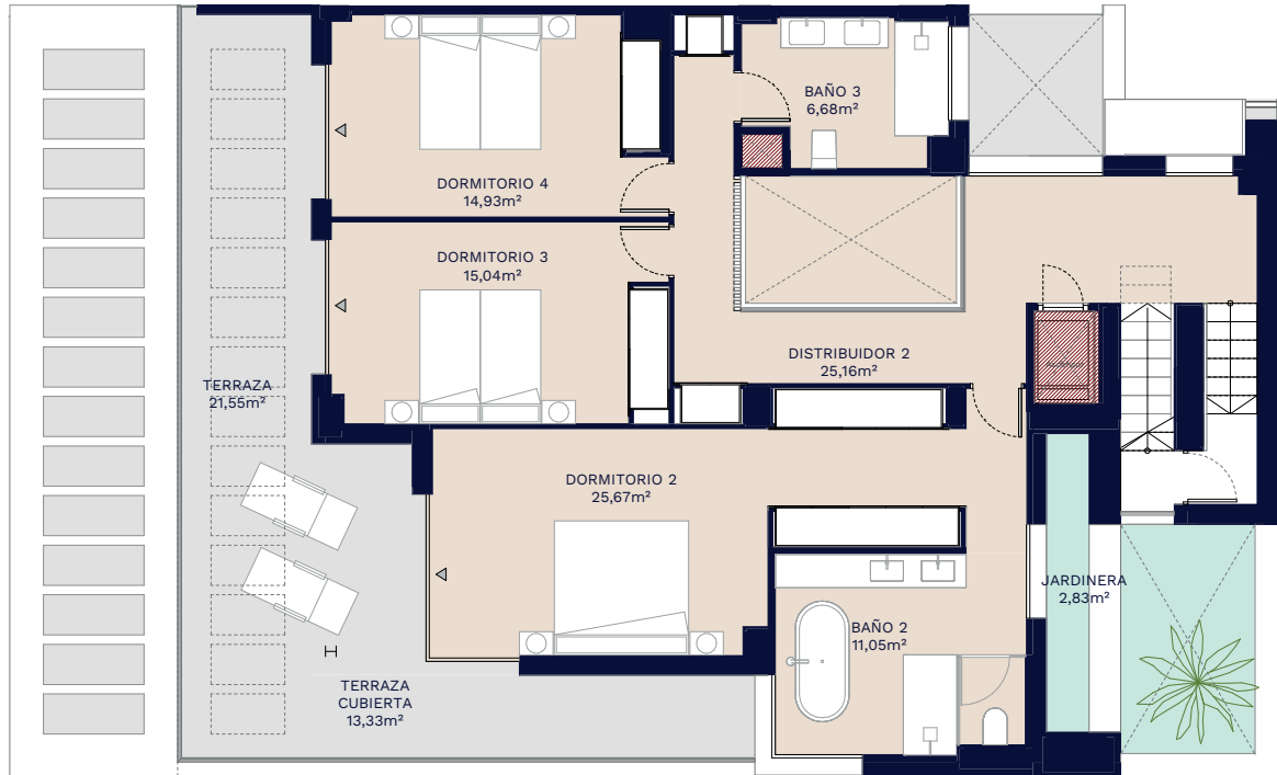
PLANTA PRIMERA
