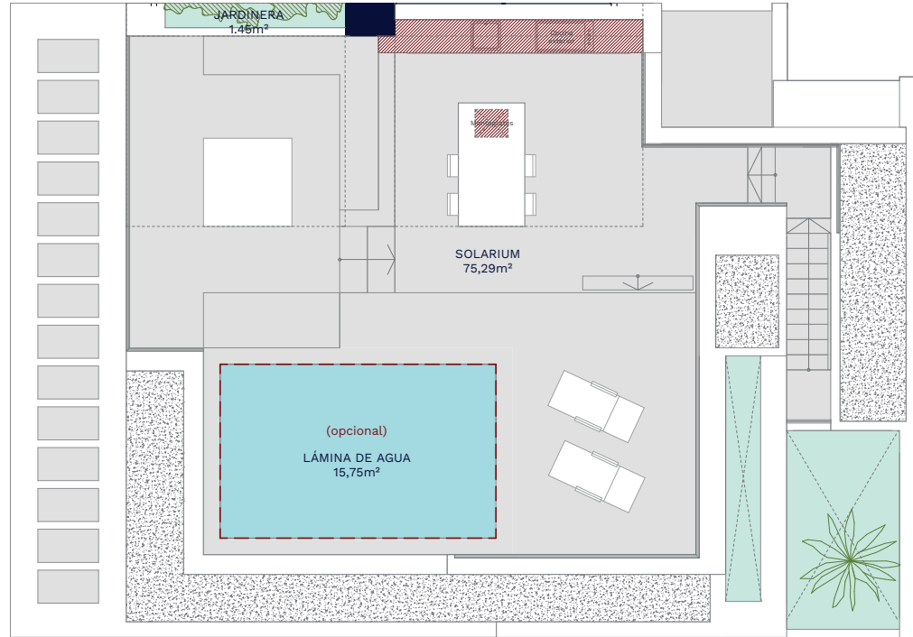
PLANTA CUBIERTA
